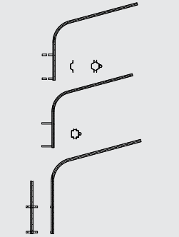
Однорожковые гнутые приставные (на хомутах)
