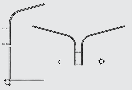
Двухрожковые гнутые приставные (на хомутах) (по ПСР)
