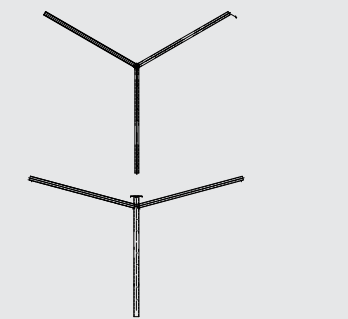
Трехрожковые сварные (на фланце) (по ОИ)
